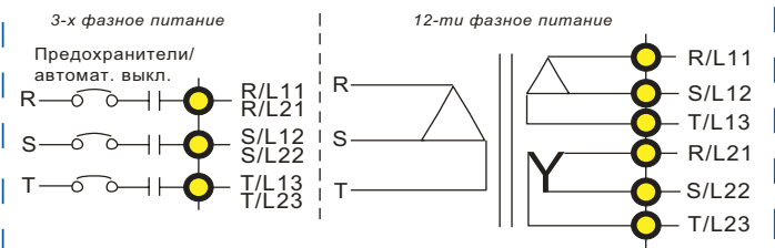
Рис.1. Входные клеммы для типоразмеров G и H
